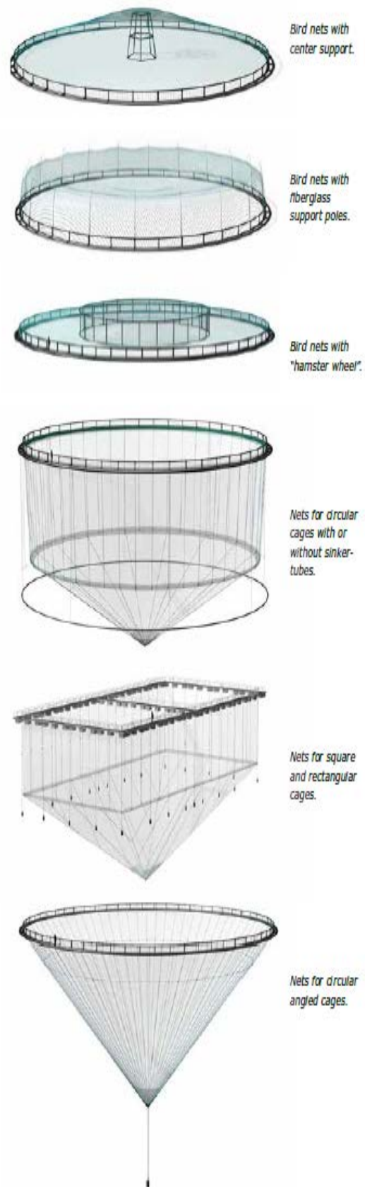
网箱主要样式
